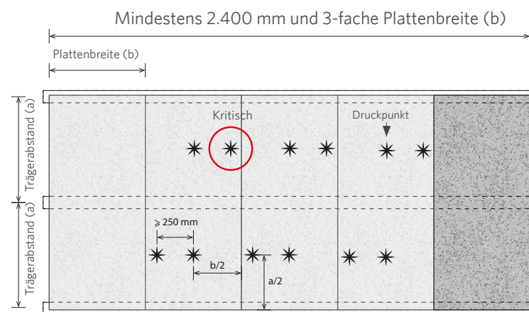
Prüfaufbau zur Bestimmung von Punktbelastungen nach EN 1195.
